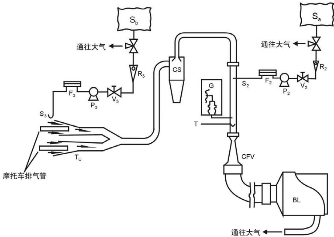
图 CB.2 排气分析系统示例 2
