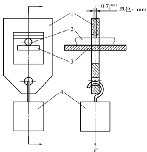
1——试验构架；2——样品；3——支架；4——砝码。
